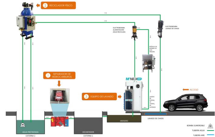
Diagrama de tratamiento de aguas – reciclador físico
