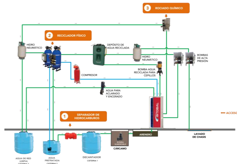
Diagrama de tratamiento de aguas – reciclador físico
